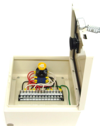
UPS からの配線は端子台へのみ
