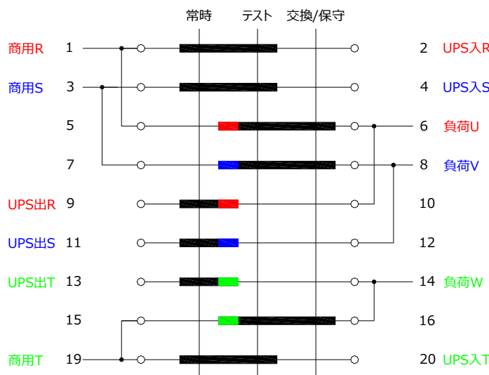
三相用 接点構成図 J-3696
