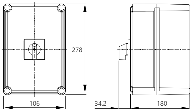
外形図 E
