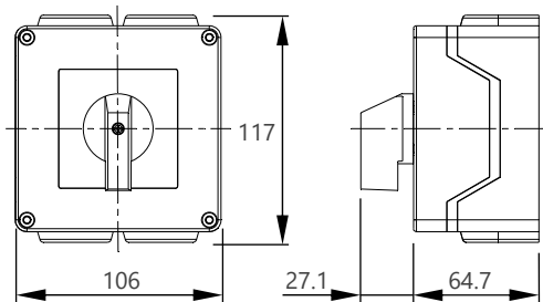
外形図 C
