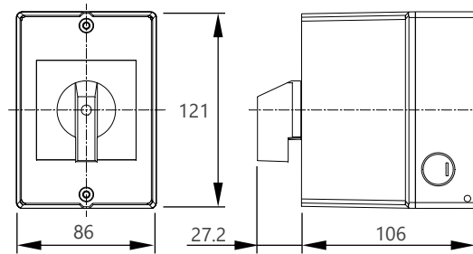
外形図 D
