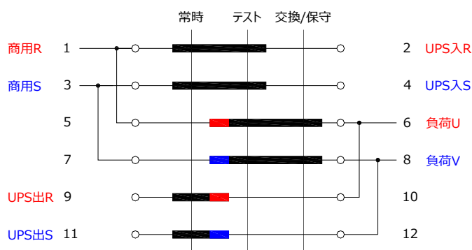
単相用 接点構成図 J-3588
