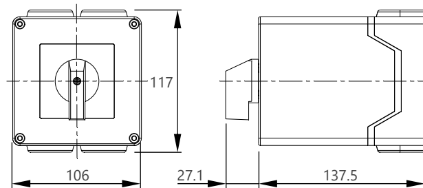
外形図 D
