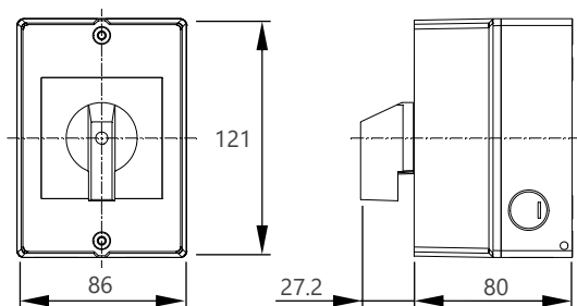
外形図 C
