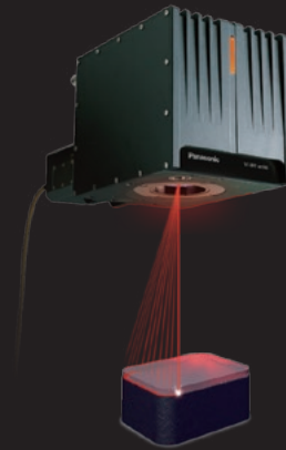
ガルバノスキャンニング式レーザー加工機
