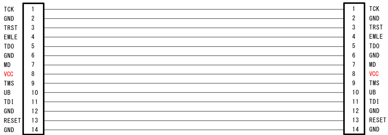
ケーブル結線図
