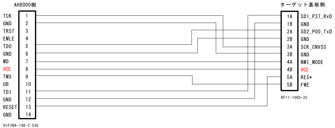
ケーブル結線図
